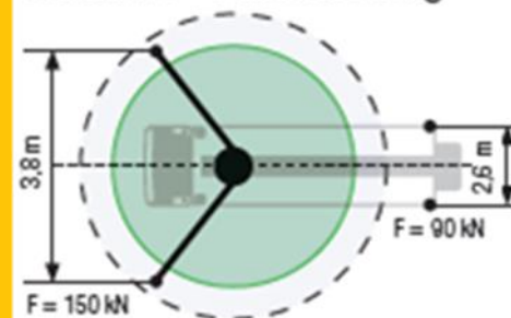
Standard – Vollabstützung
